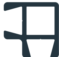
Pfostenmaße P60/E Ecke 60x60 mm
